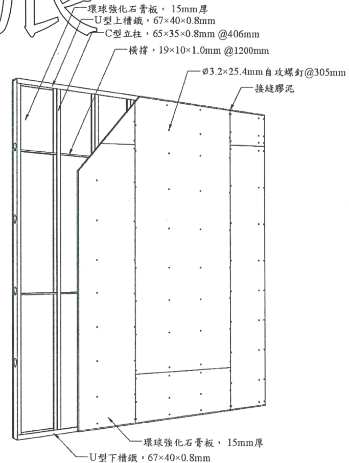
透視示意圖
