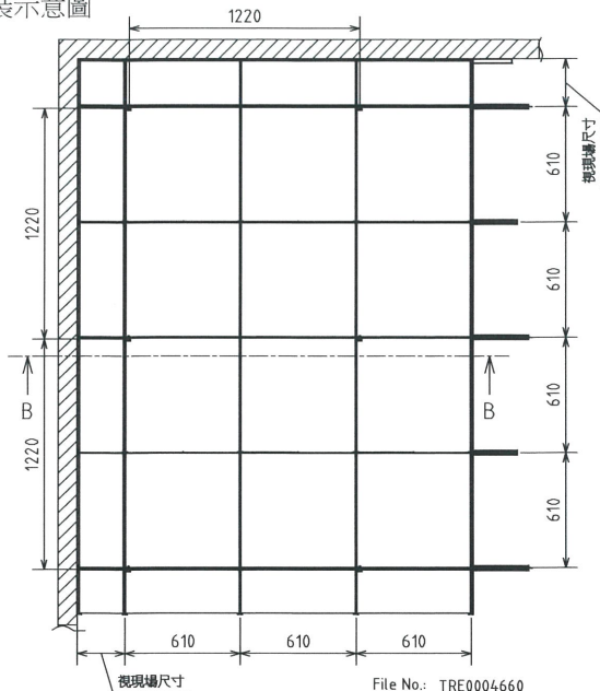
平面組裝示意圖
