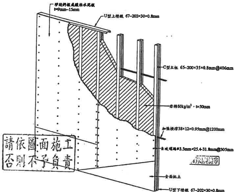
圖 1 立面示意圖 單位:mm
