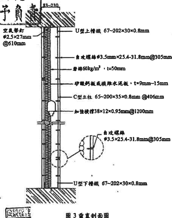
圖 3 垂直剖面圖 單位:mm
