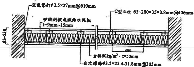
圖 2 水平剖面圖 單位:mm
