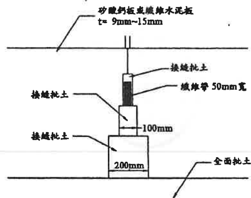
圖 4 接縫施工圖 單位:mm
