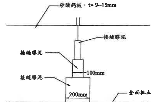
圖 4 接縫施工圖 單位:mm
