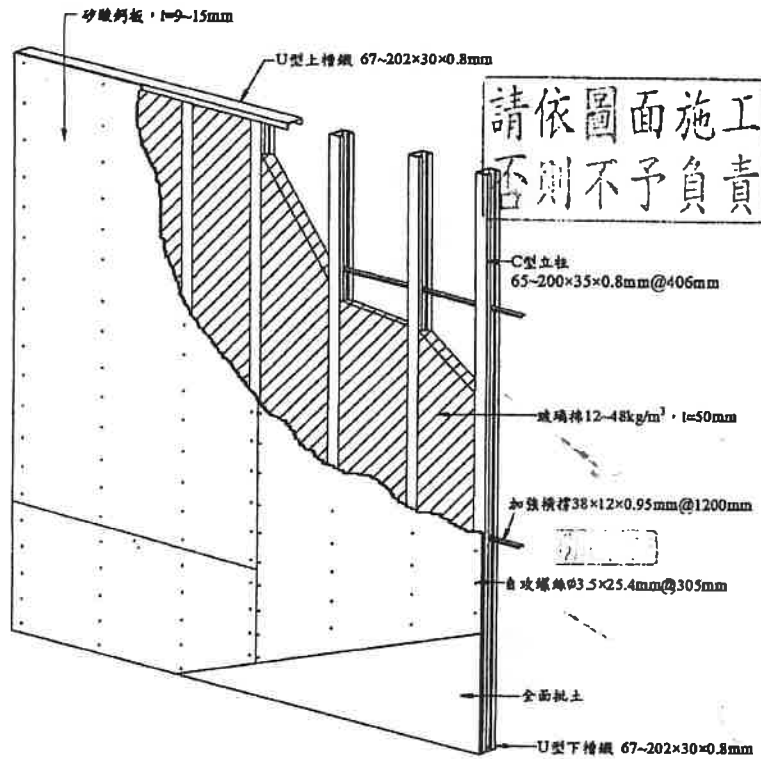
圖 1 立面示意圖 單位:mm
