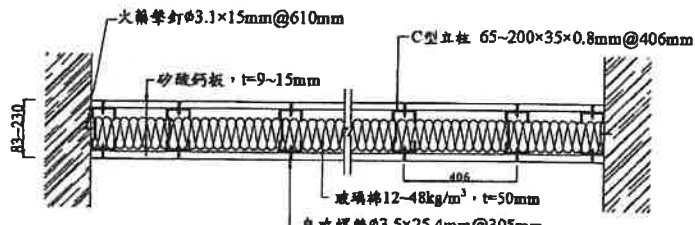
圖 2 水平剖面圖 單位:mm
