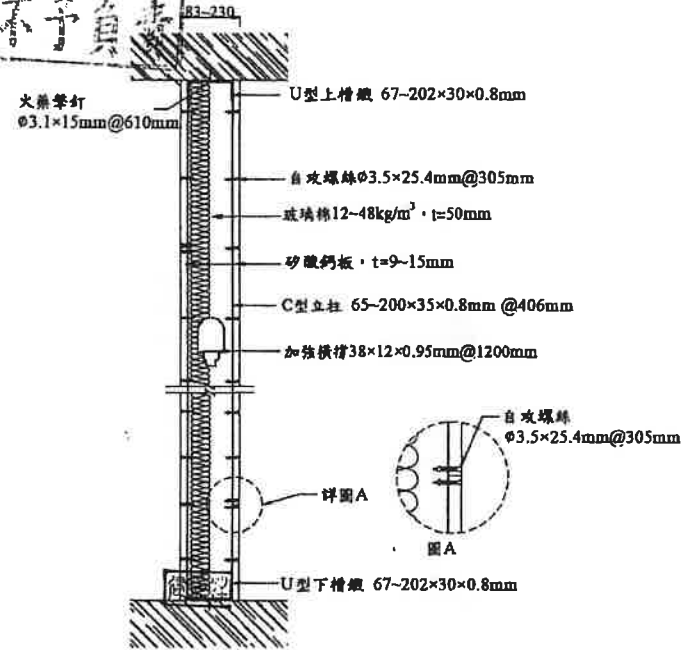
圖 3 垂直剖面圖 單位:mm
