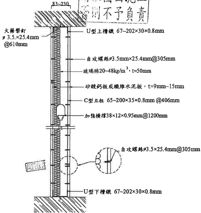
圖 2 垂直剖面圖 單位:mm
