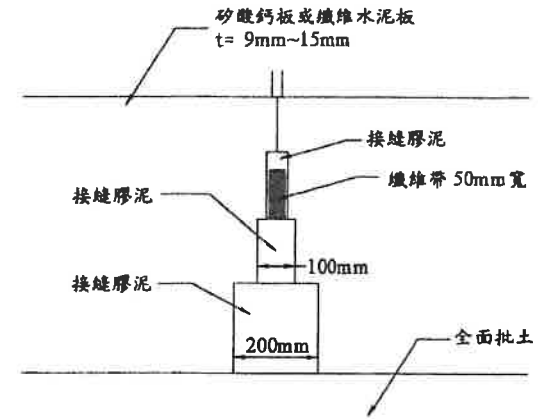
圖 4 接縫施工圖 單位:mm
