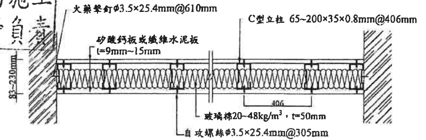
圖 3 水平剖面圖 單位:mm
